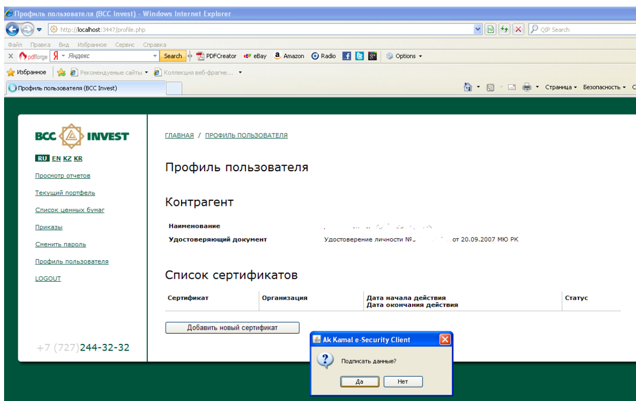
Рис 21. Активация ЭЦП
