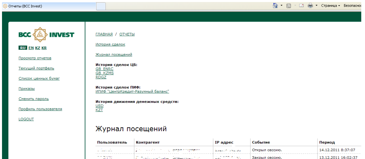
Рис 3. Журнал посещений
